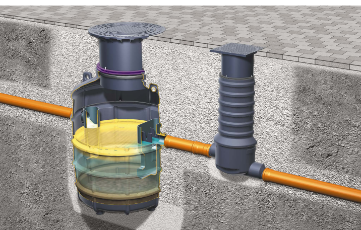
EasyClean ground (NS 2 - NS 6): for utendørs nedgravd installasjon
