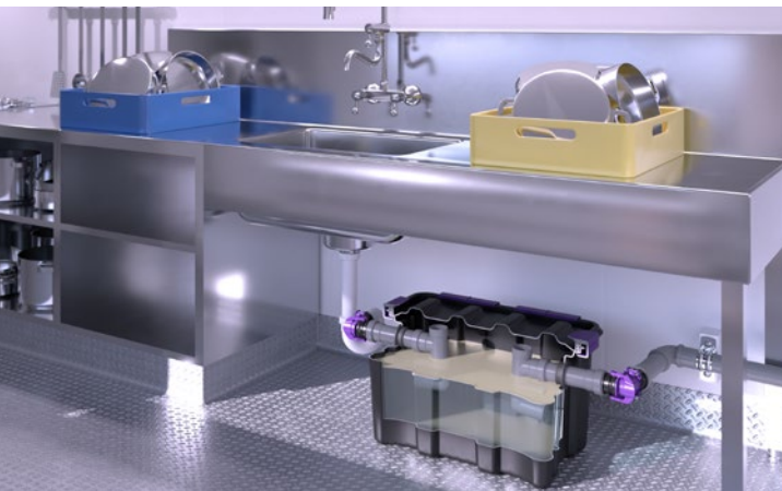
EasyClean free UnderSINK (NS 0.7): for frittstående innendørs installasjon der plassen er meget begrenset
