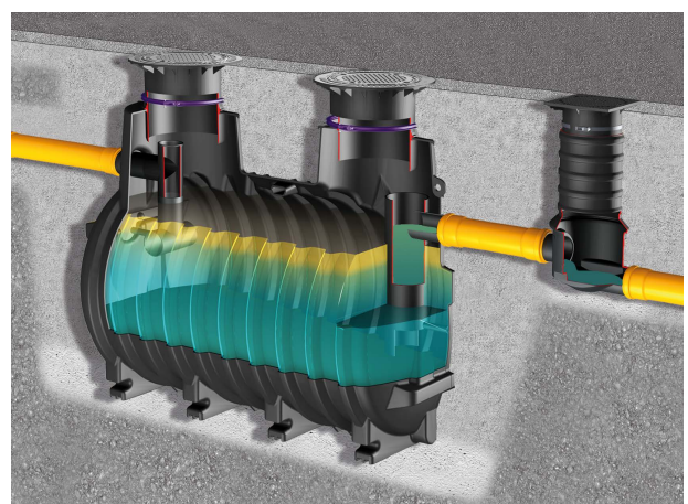
EasyClean ground (NS 10 - NS 35): for utendørs nedgravd installasjon
